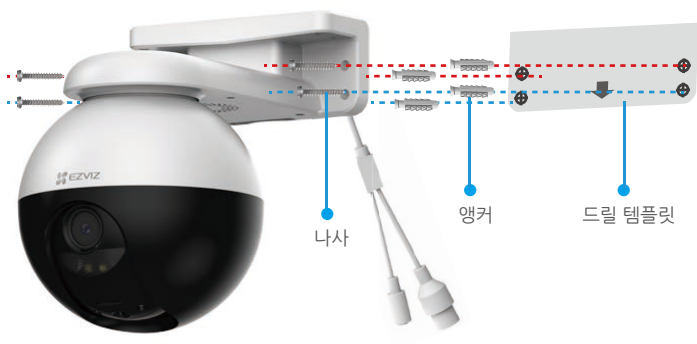
그림 2 벽 장착
